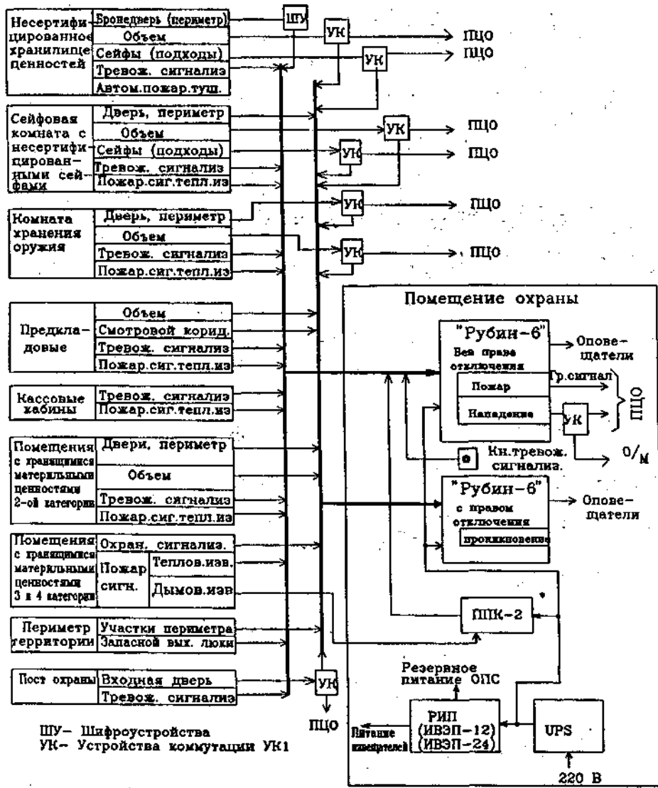
Рис.1. Примерная структурная схема оборудованная объекта средствами ОПС на базе прибора "Рубин-6" по варианту 1.
