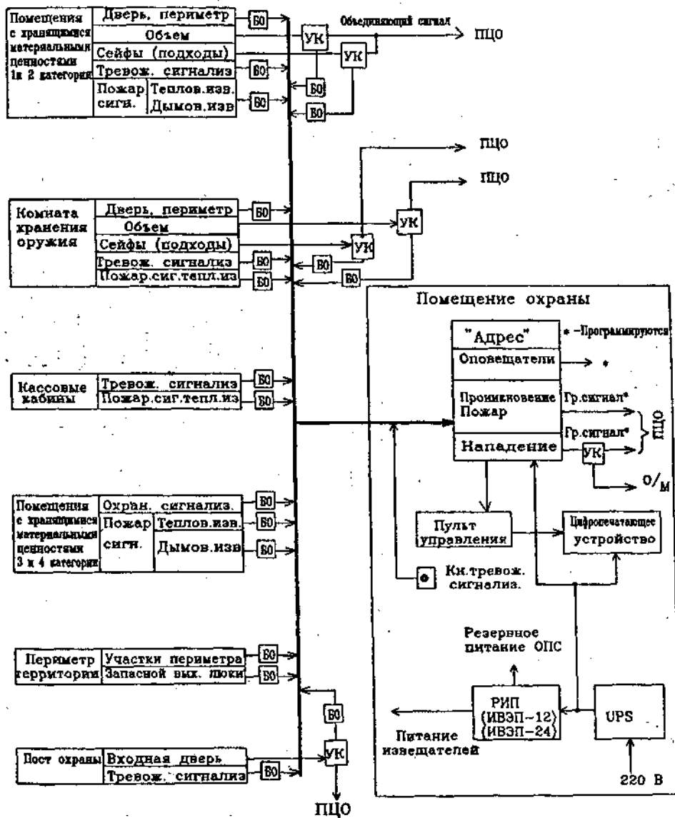
Рис.4. Примерная структурная схема оборудования объекта средствами ОПС на базе прибора "Адрес" по варианту 2.
