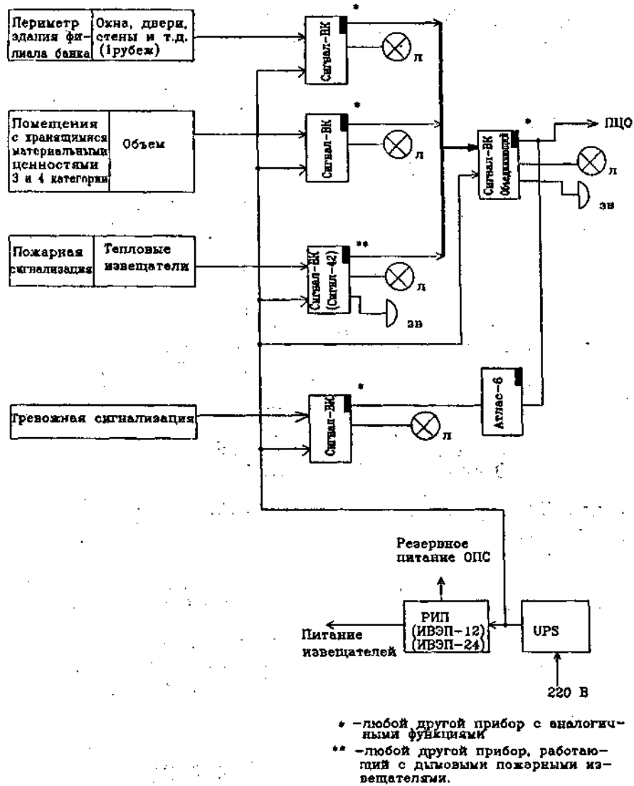
Рис.9. Примерная структурная схема оборудования объекта средствами ОПС на базе приемно-контрольного прибора "Сигнал-ВК" и системы уплотнения "Атлас-6" по варианту 7.
