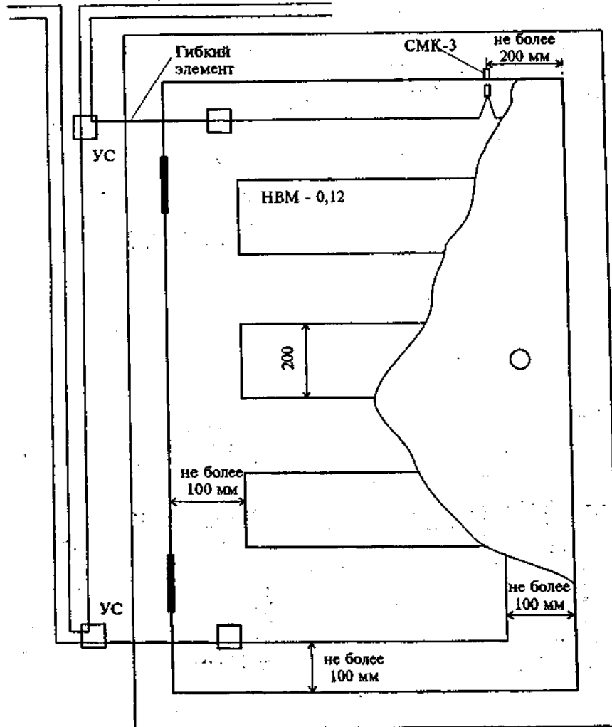
Рис. 3 Блокировка дверей (ворот) на открывание и пролом проводом НВМ и извещателями магнитоконтактными (выключателями конечными)
