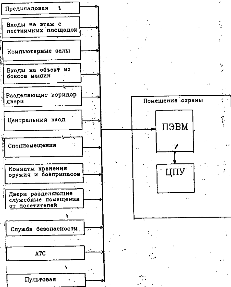
Рис.1. Примерная структурная схема оборудования объекта системой контроля доступа.
