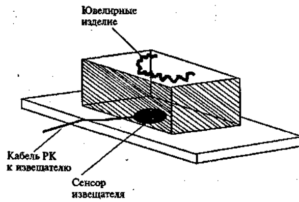
Рис.8. Блокировка отдельных предметов извещателем поверхностным пьезоэлектрическим "Гюрза-050"
