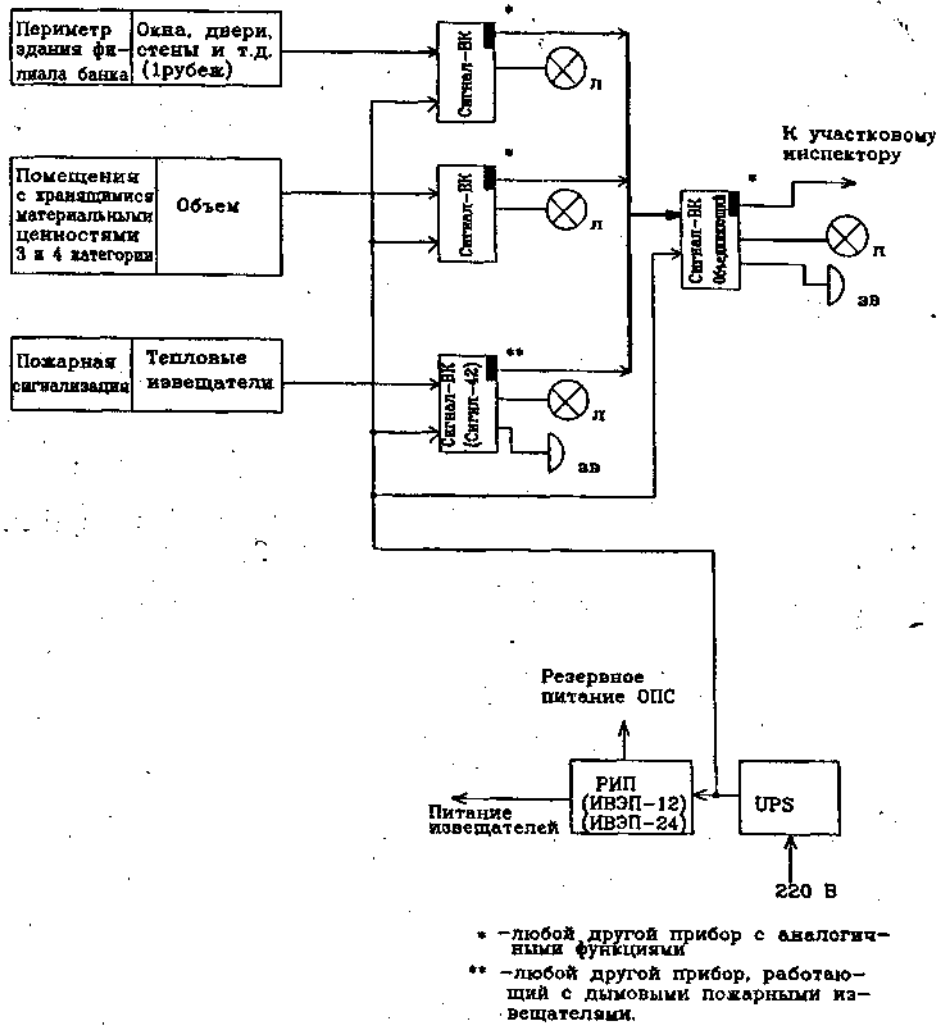
Рис.10. Примерная структурная схема оборудования объекта средствами ОПС на базе приемно-контрольного прибора "Сигнал-ВК" по варианту В.
