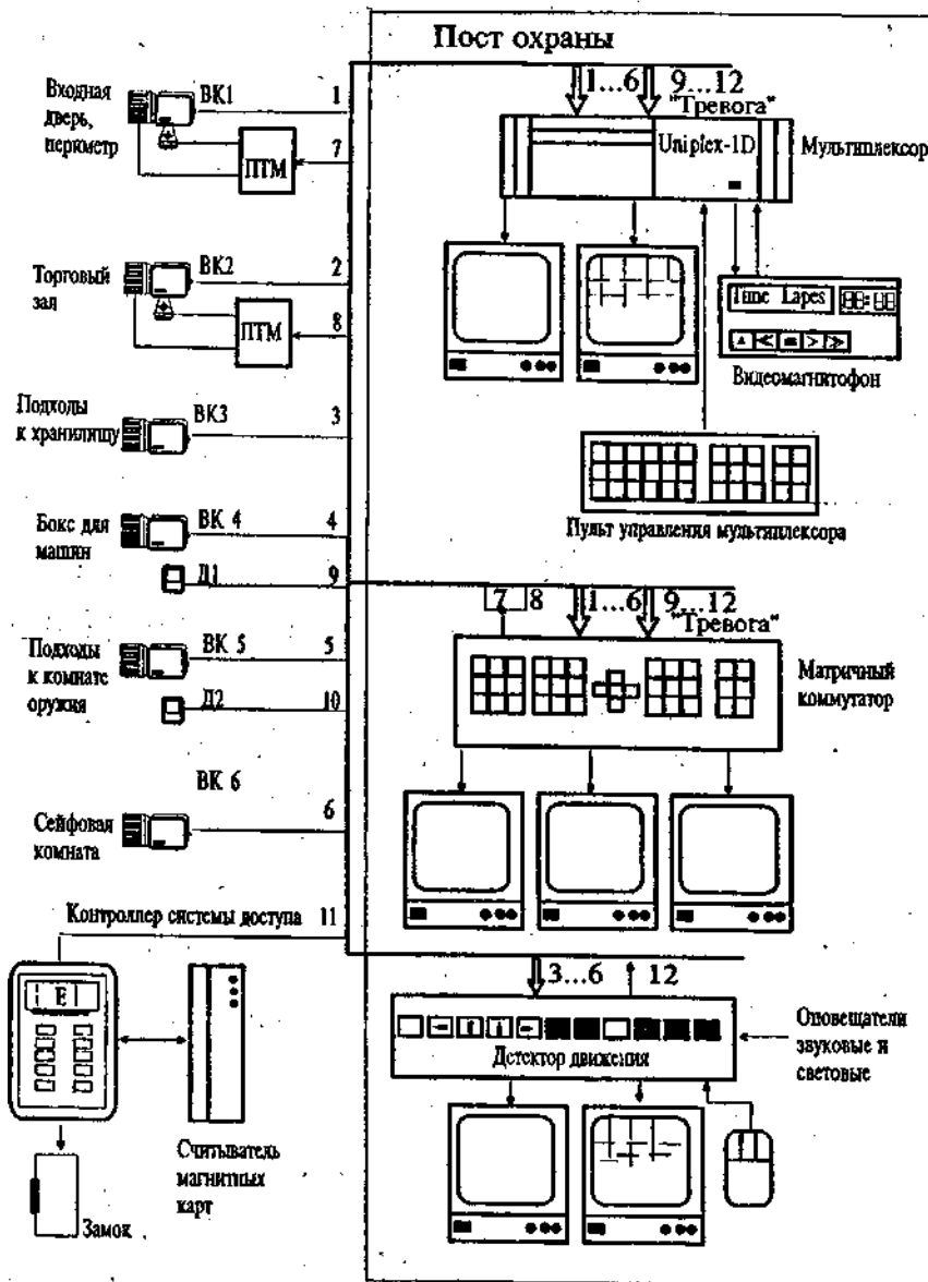
Рис.2. Примерная структурная схема оборудования объекта системой видеоконтроля.
