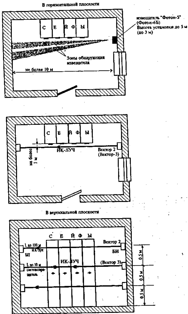
Рис.13. Блокировка сейфа (предметов) извещателями оптико-электронными
