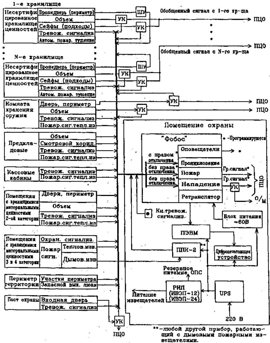
Рис.3. Примерная структурная схема оборудования объекта, имеющего несколько хранилищ, на базе СПИ "Фобос" по варианту 1.
