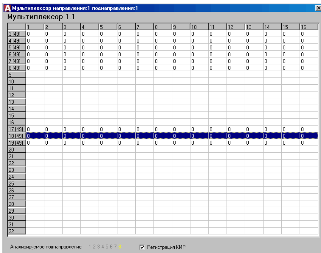
Рисунок 14 – Окно Мультиплексора.
